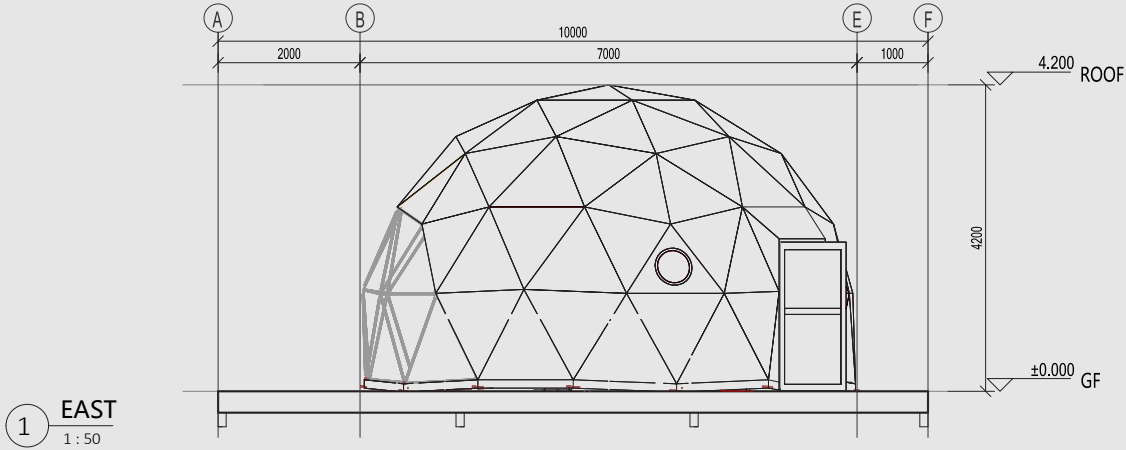
Elevation
